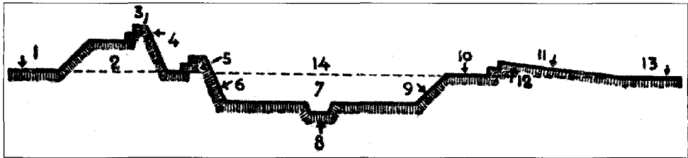
Afb. 4 Profiel. 1 Terreplein (binnenruimte der vesting) 8 Cunette. 2 Hoofdwal 9 Contrescarptalud 3 Borstwering 10 Bedekte weg 4 Escarptaluds 11 Glacis 5 Onderwal 12 Contrescarp 6 Escarptaluds 13 Maaiveld 7 Gracht 14 Horizontale meetlijn
